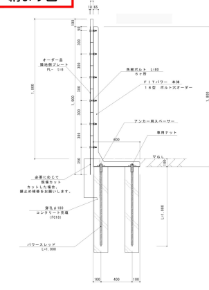
納まり図
