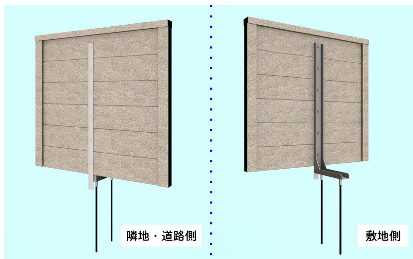
納まり図
