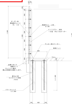
納まり図
