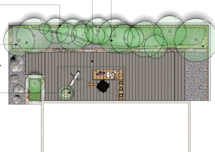
ガーデンルームGf デッキ仕様 2.0間×6尺 H22 正面開口 腰壁+高窓・テラスサッシ 左側面開口 折戸 左側面開口 腰壁+高窓 スタイルシェード 照明 ビームラインライト
