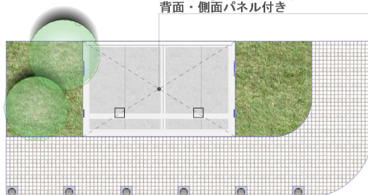
アーキラインシェルター GK-A型 W25-40型 柱H:2100 色：ナチュラルシルバー 屋根材：強化合わせガラス 背面・側面パネル付き
